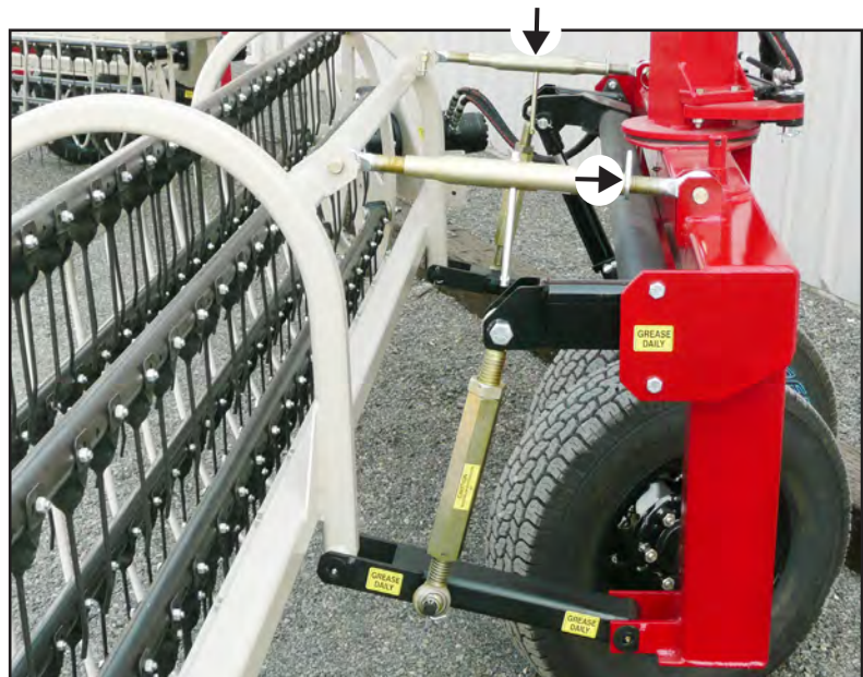
Fig. 16 BASKET TILT
